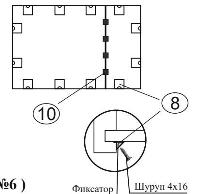
СХЕМА РАСПОЛОЖЕНИЯ ФИКСАТОРОВ
