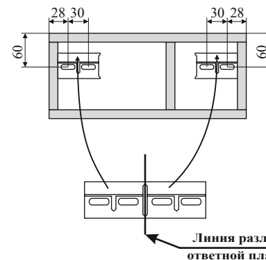
СХЕМА КРЕПЛЕНИЯ ОТВЕТНЫХ ПЛАНК К СТЕНЕ ( рис. №5 )
