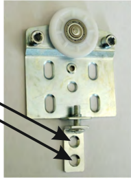
Ходовой ролик внутренней двери.
