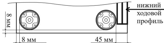
СХЕМА ПРИСАДКИ ОПОР-НОГ
