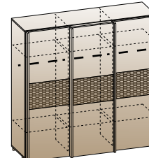
КП-231 2172x1792x650
